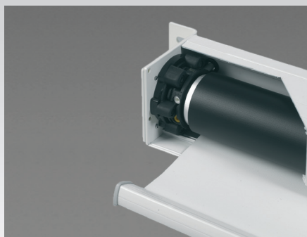
Geräuschloser Motorantrieb durch Spezialmotor mit Gummilager.
